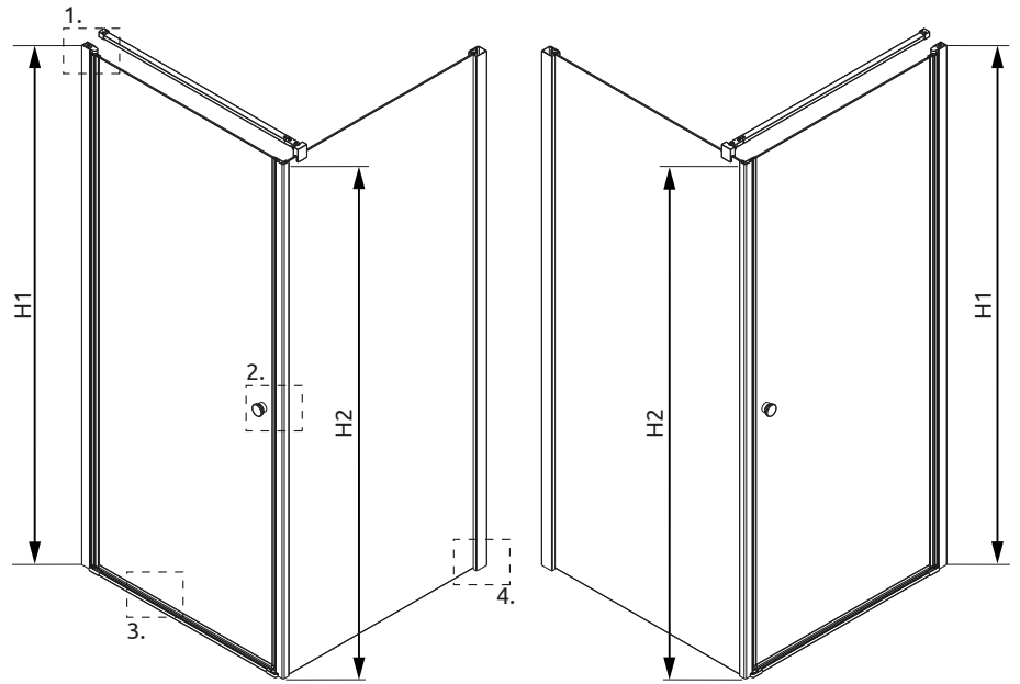
Lavostranný sprchovací kút Variant L
