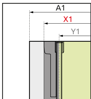
Lavostranný sprchovací kút Variant L
