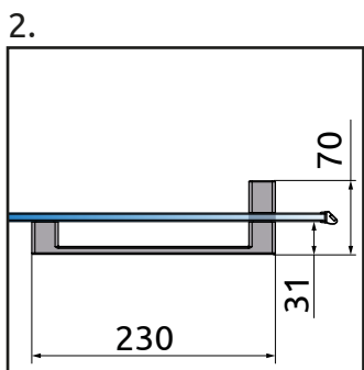
Lavostranný sprchovací kút Variant L
