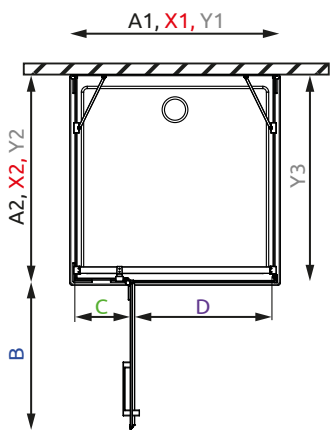
Lavostranný sprchovací kút Variant L
