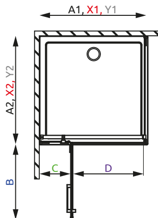
Lavostranný sprchovací kút Variant L
