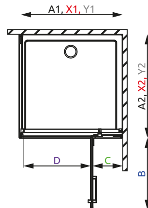
Pravostranný sprchovací kút Variant R
