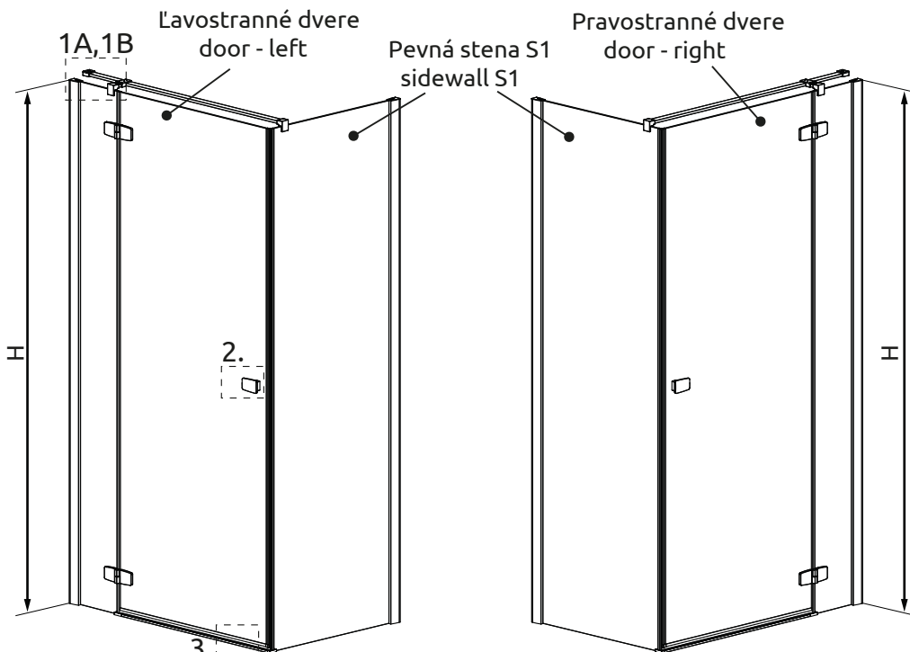
Lavostranný sprchovací kút Variant L
