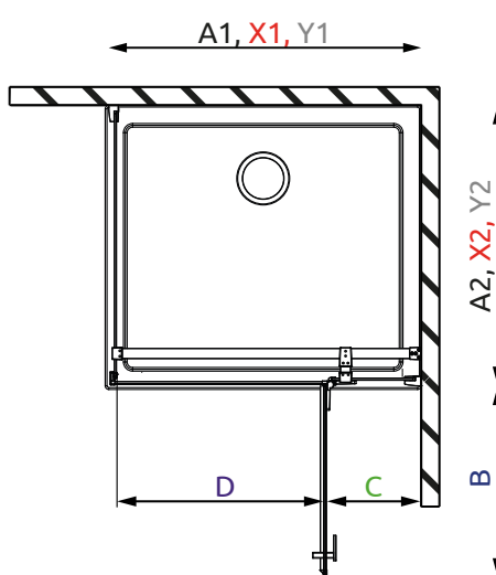
Pravostranný sprchovací kút Variant R
