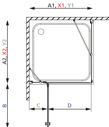
Ľavostranný sprchovací kút Variant L
