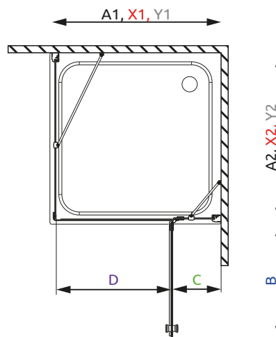
Pravostranný sprchovací kút Variant R
